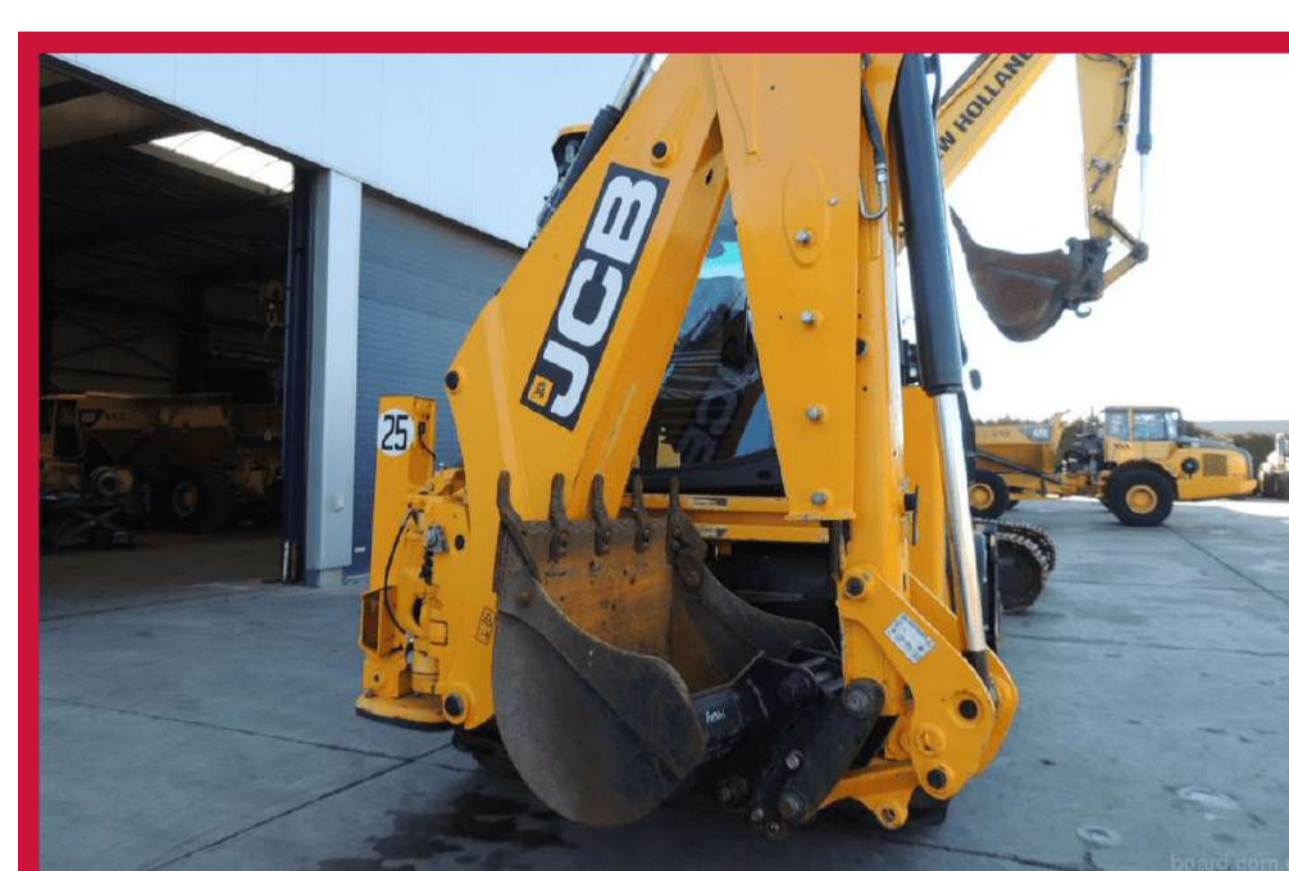
Отверстия в стреле погрузчика
