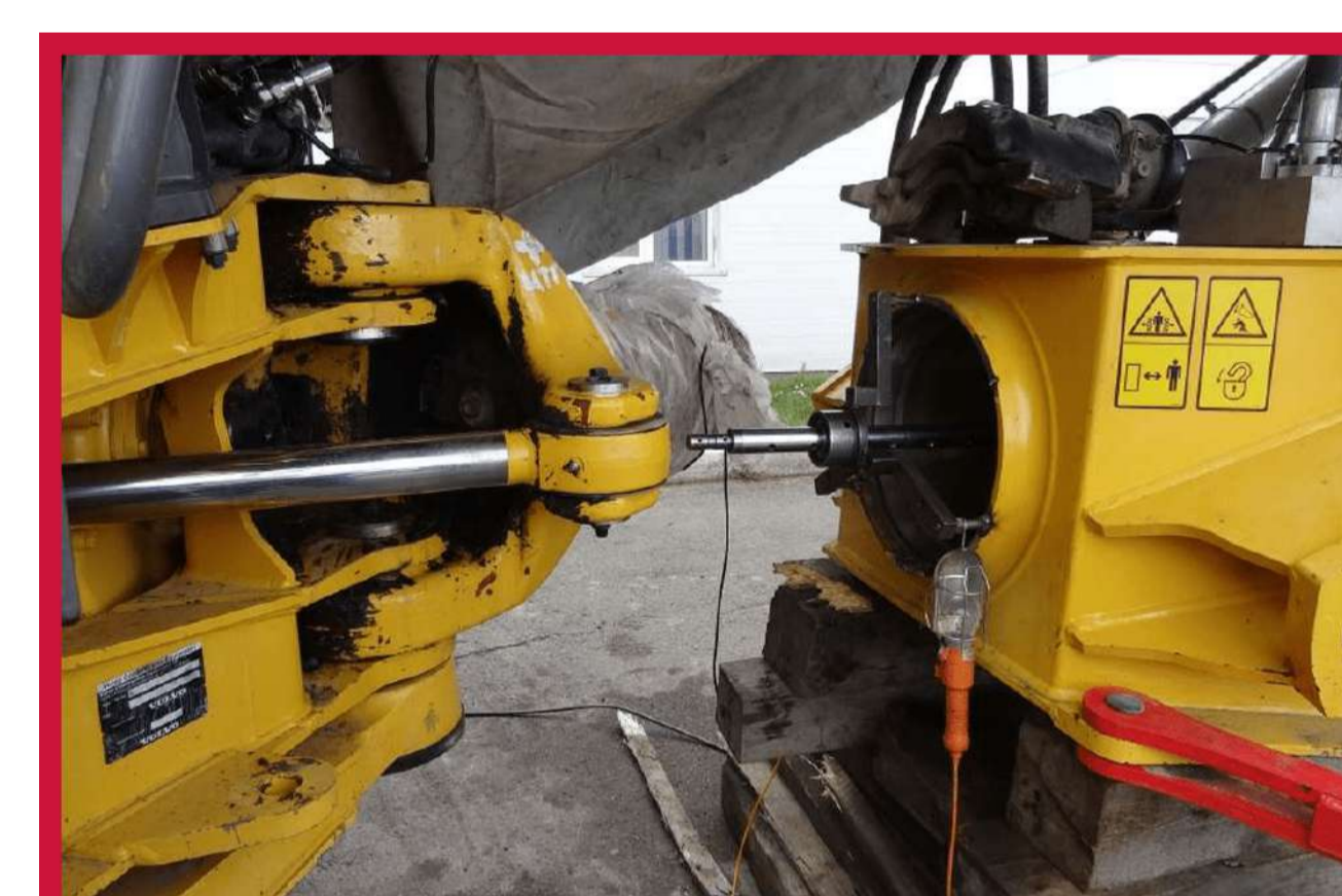
Отверстия шарнирного соединения полурам спецтехники
